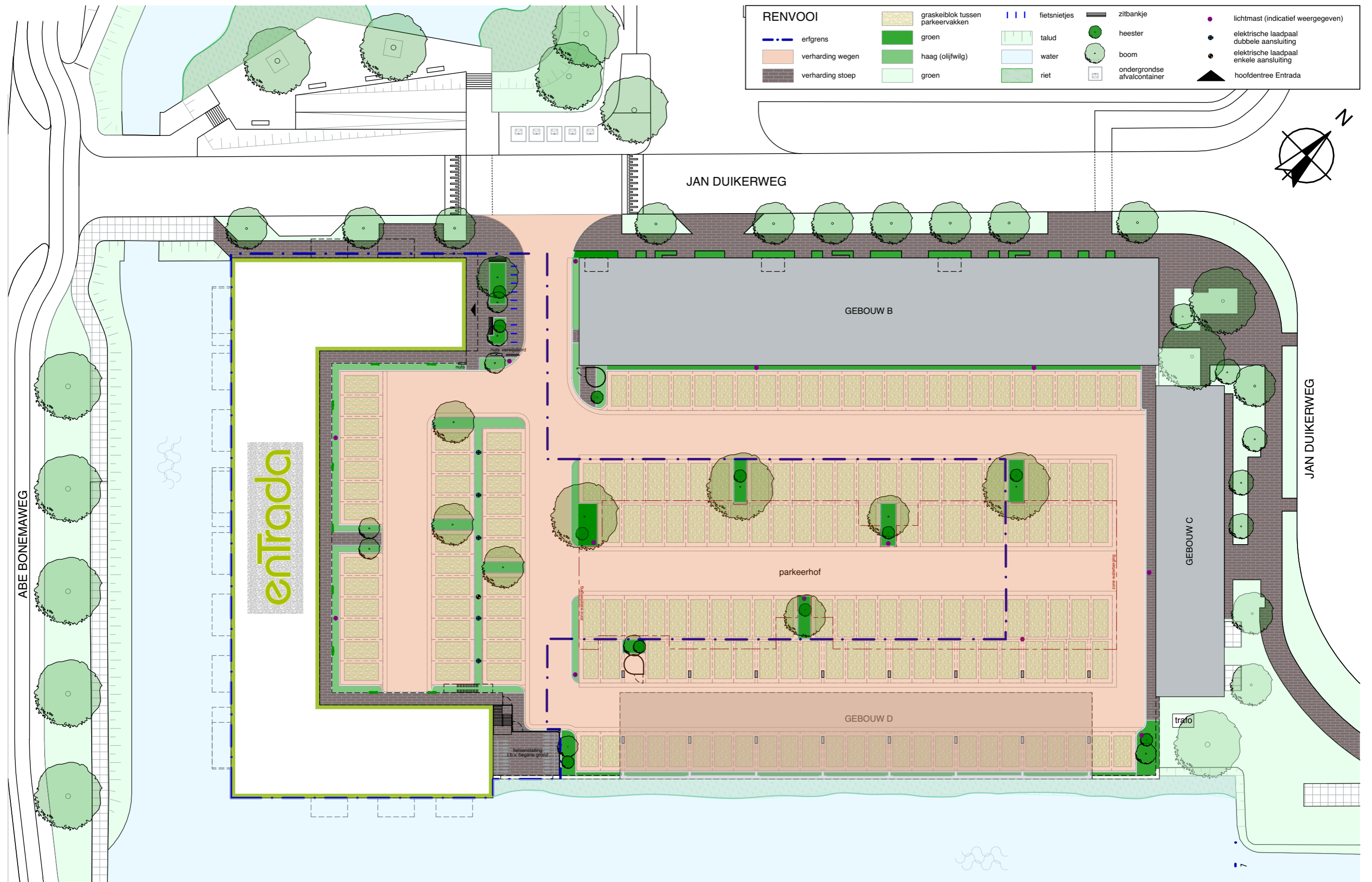
Situatietekening
